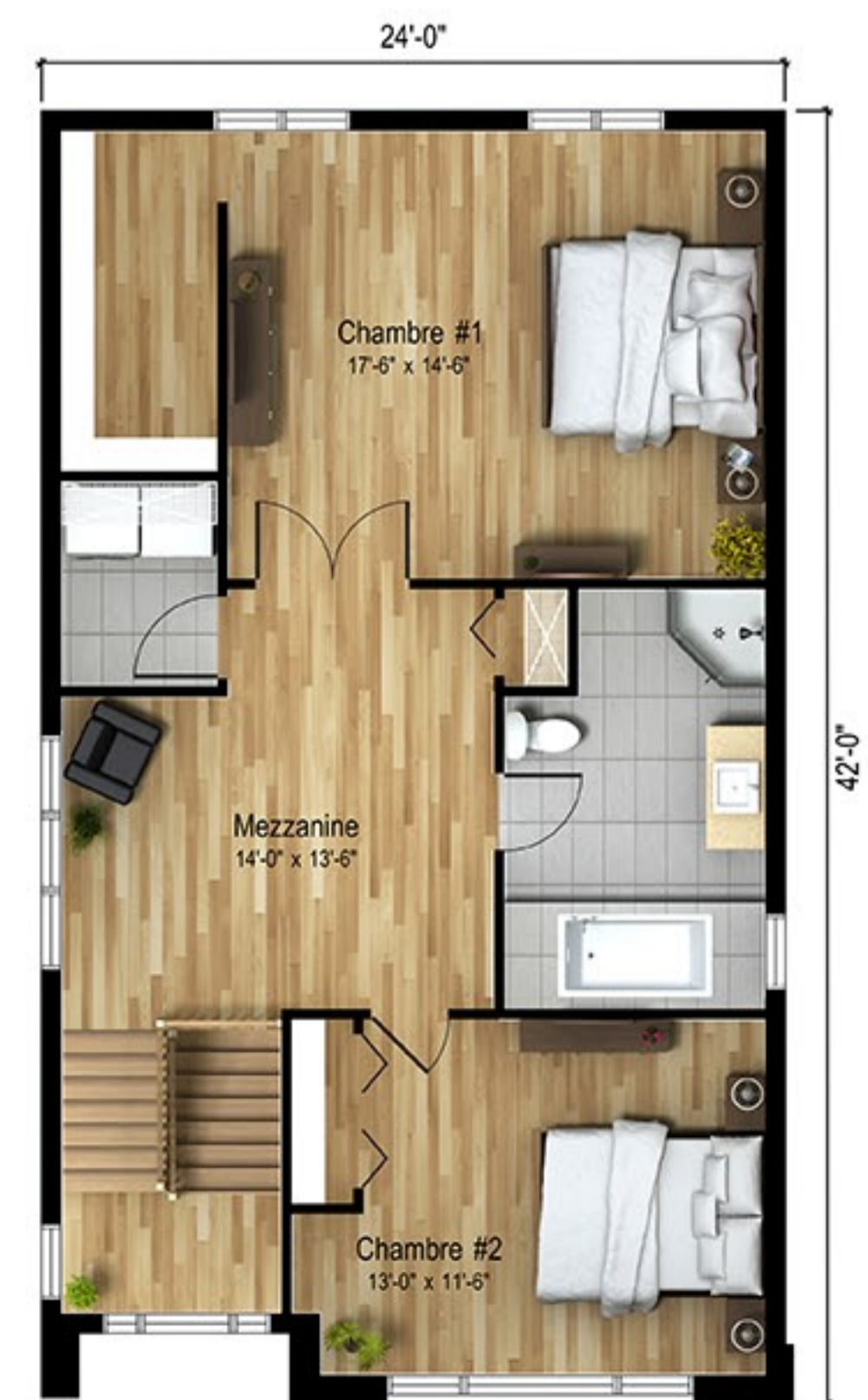
Étage Option 2 Sup. Habitable: 988 pi 2 Sup. Totale: 1678 pi 2
